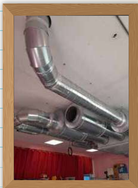
Mise en place d'une VMC double flux pour une amélioration de la qualité de l'air dans les locaux scolaires
